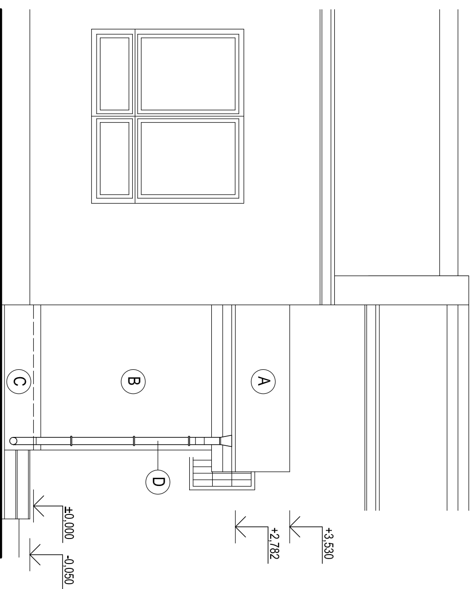
POHLAD VÝCHODNÝ M=1:50
